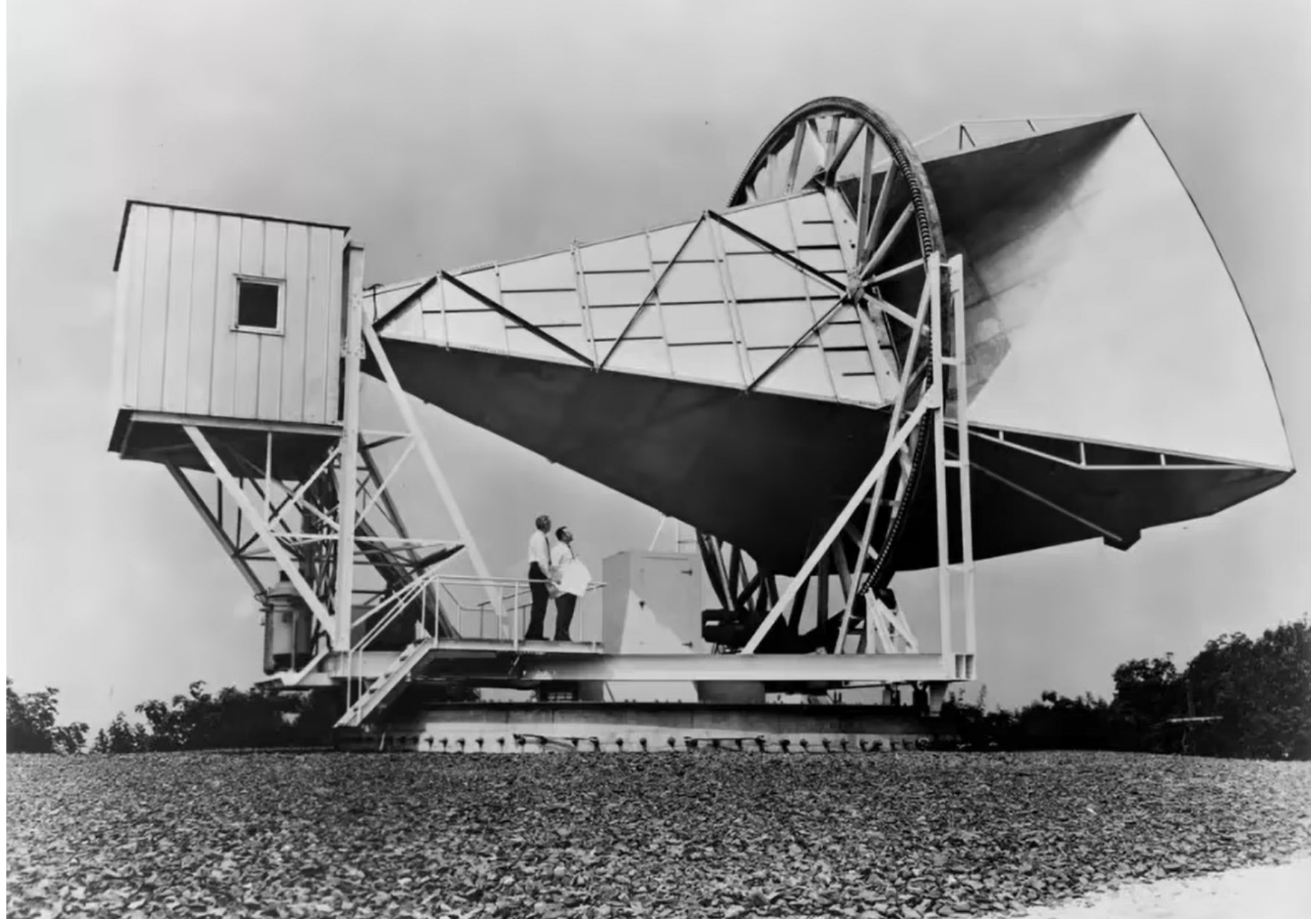
1962. Un'antenna a corno di Hogg fotografata nel New Jersey. Serve a trasmettere e ricevere su micro-onde canali televisivi o chiamate telefoniche (anche decine di migliaia contemporaneamente).
